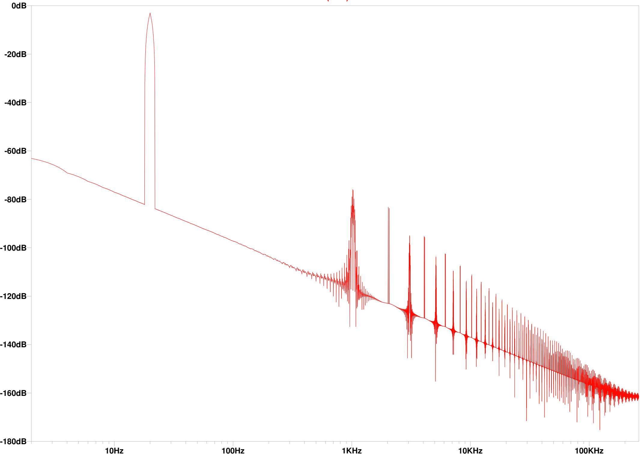
V(vout)
