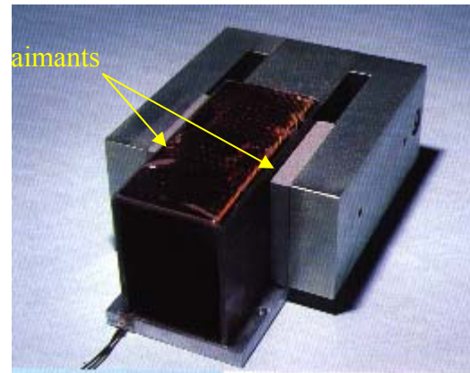
Actionneur à bobine mobile (ETEL) (type haut parleur)
