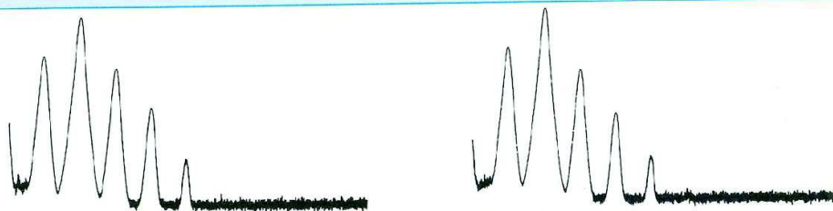
Fig. 3 : Les deux spectres de distortion pour V_{out} = 3V (à gauche avec l'atténuateur, à droite avec le filtre).
