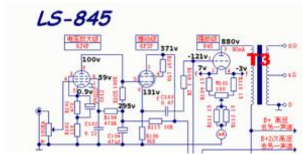
Schéma LS 845 Liang
