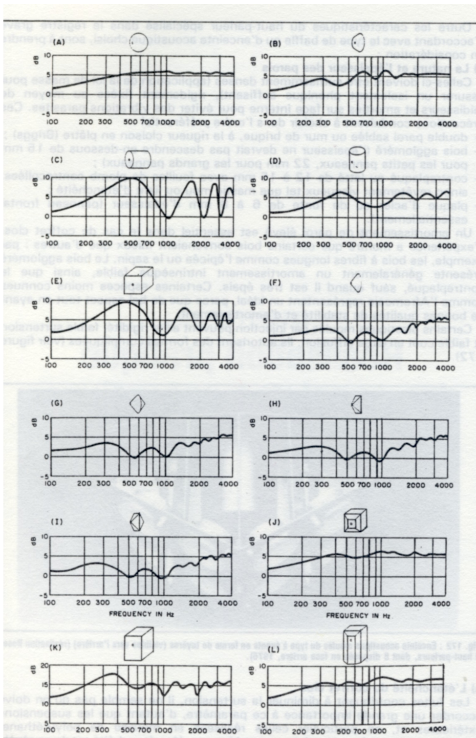
Fig. 173 : Influence de la forme de l'enceinte acoustique sur la réponse du haut-parleur (d'après H.F. Olson).
