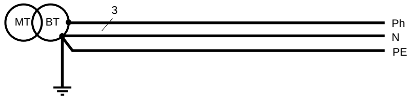
c - SLT TN-S
