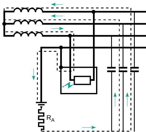
Fig. 8 : schéma IT.
