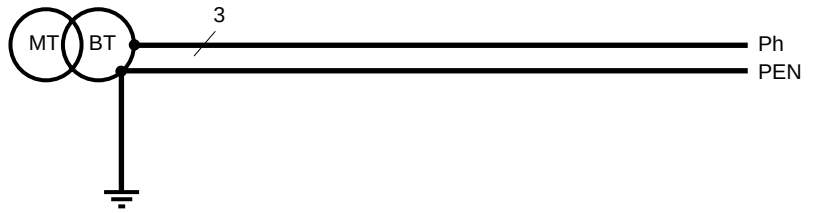
a - SLT TN-C
