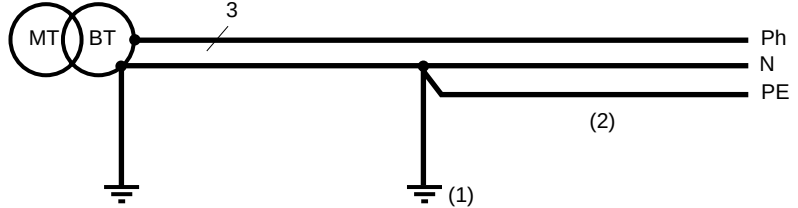
b - SLT TN-C-S
