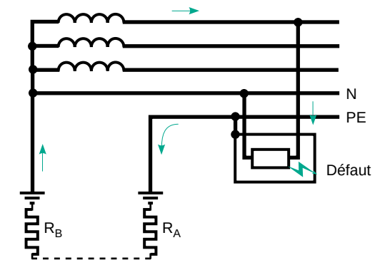
Fig. 7 : schéma TT.
