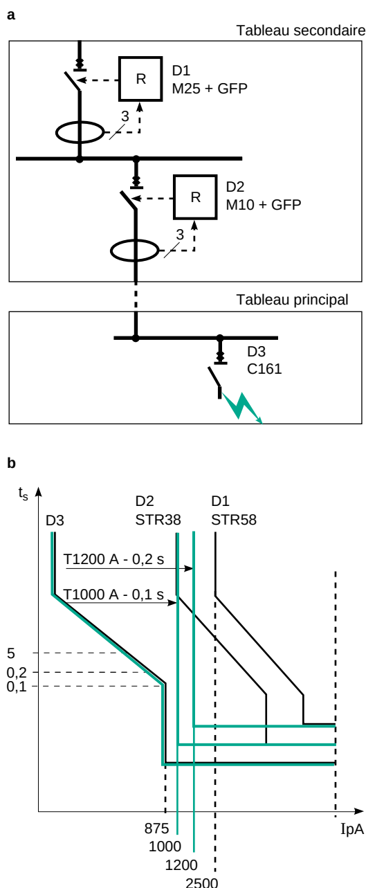
Fig. 17 : sélectivité entre protection contre les courts-circuits aval (D3) et protections de terre (GPF) amont, en vert.
