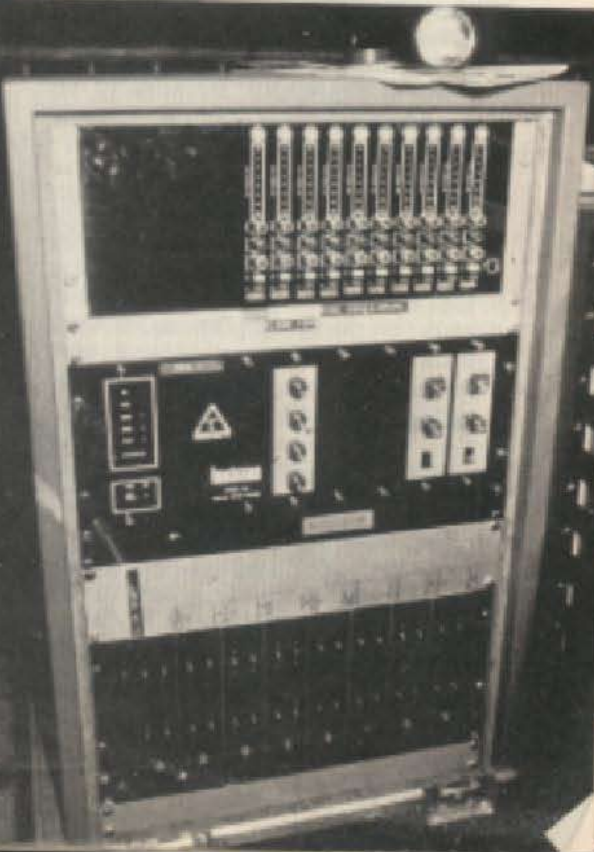
15) Rack technique: les noises / gates Kepex, le générateur digital de retard Lexicon et les sus-penseurs de bruits de fond DBX.
