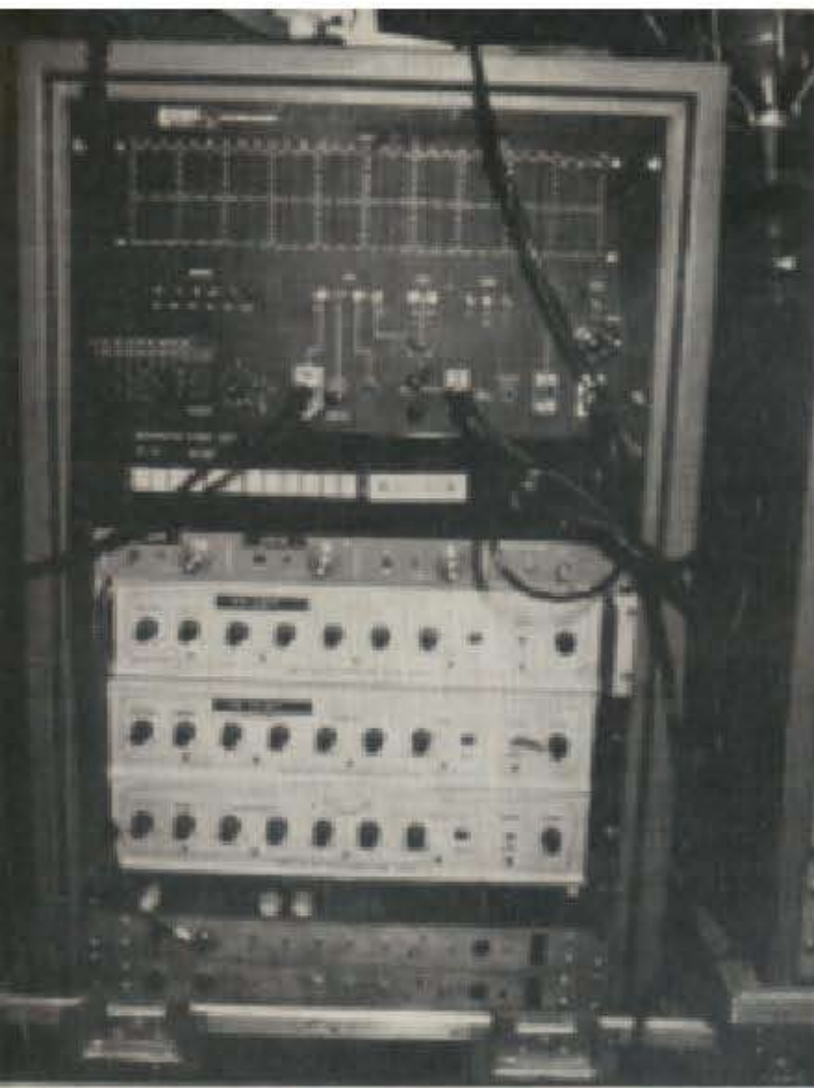
11) Rack technique : 5 générateurs de phasing et en haut l'analyseur de spectre en temps réel.
