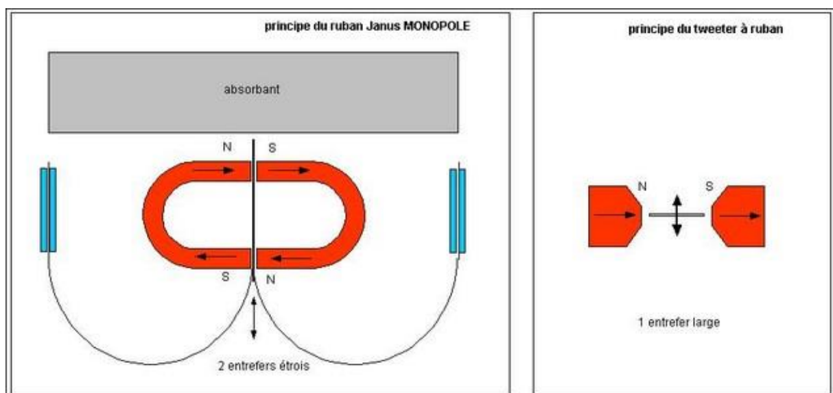
Schéma de montage :
